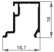
AG-057 0,167 Kg/m
