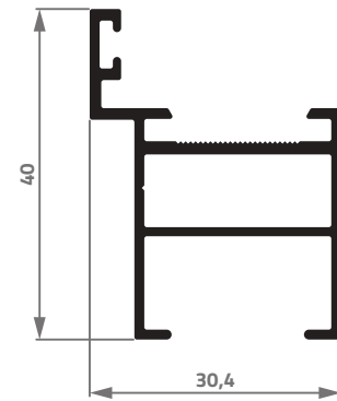
25540 0,472 Kg/m
