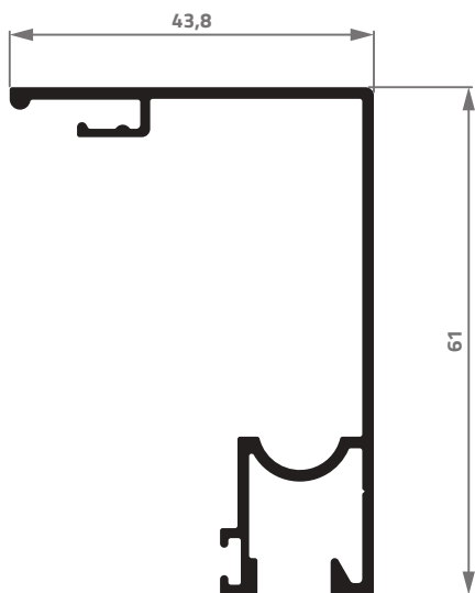
2910-L 0,632 Kg/m
