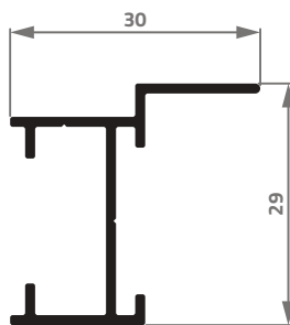
AS-071 0,277 Kg/m
