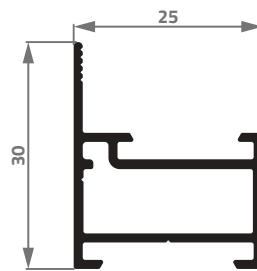
AS-080 0,355 Kg/m
