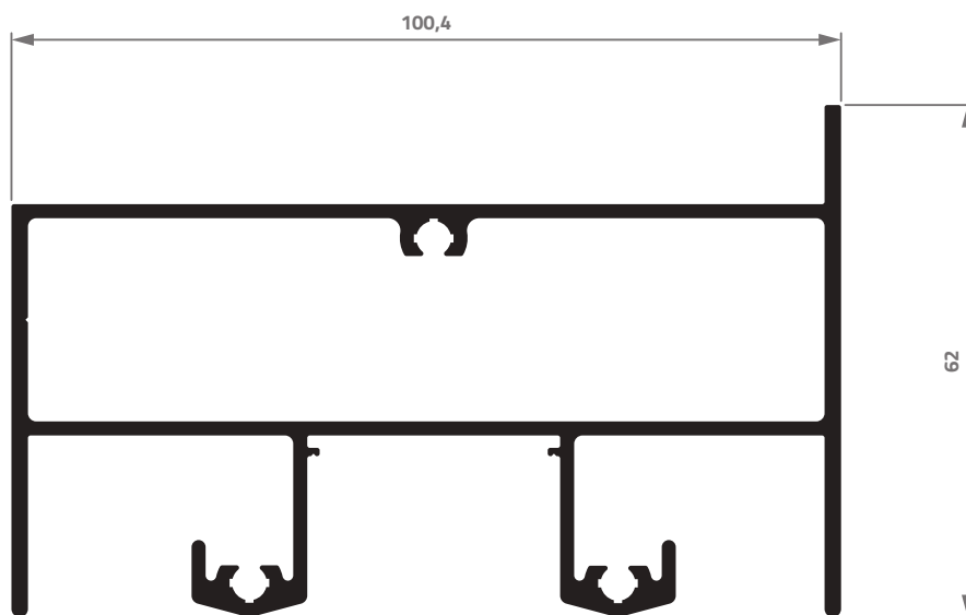
AG-004 2,035 Kg/m
