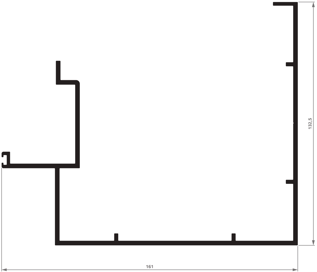
PC-601 2,979 Kg/m
