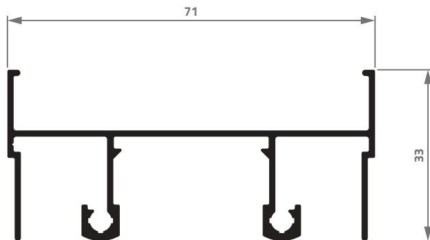
AS-001 0,713 Kg/m
