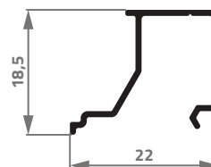
AS-103 0,141 Kg/m
