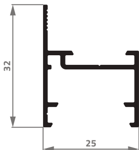
AS-088 0,292 Kg/m
