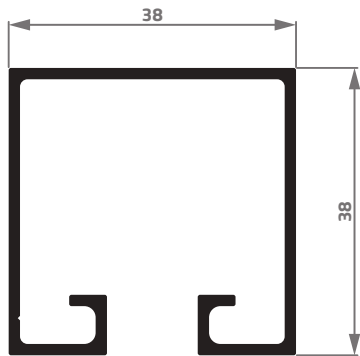
DS-314 0,737 Kg/m
