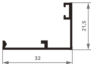
AL-026 0,227 Kg/m
