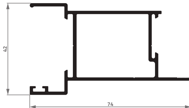
AG-051 0,916 Kg/m
