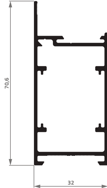
AG-043 0,935 Kg/m
