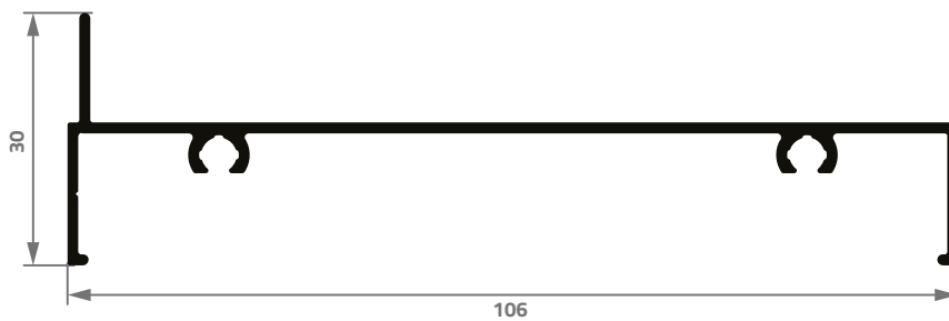
AS-018 0,630 Kg/m
