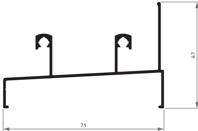
AS-002 0,650 Kg/m
