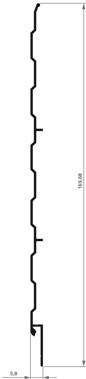
LB-001 0,626 Kg/m
