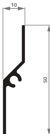
DV-113 0,253 Kg/m
