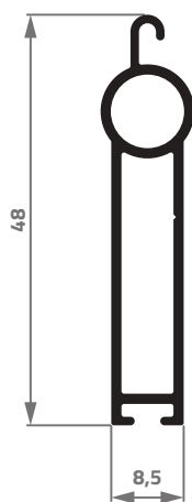
MN-055 0,366 Kg/m
