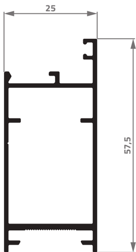
25542 0,601 Kg/m
