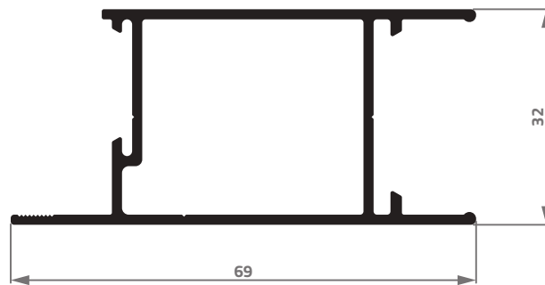
AG-050 0,817 Kg/m
