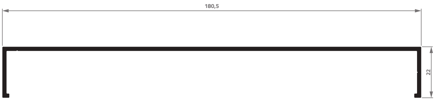
AG-035 1,089 Kg/m
