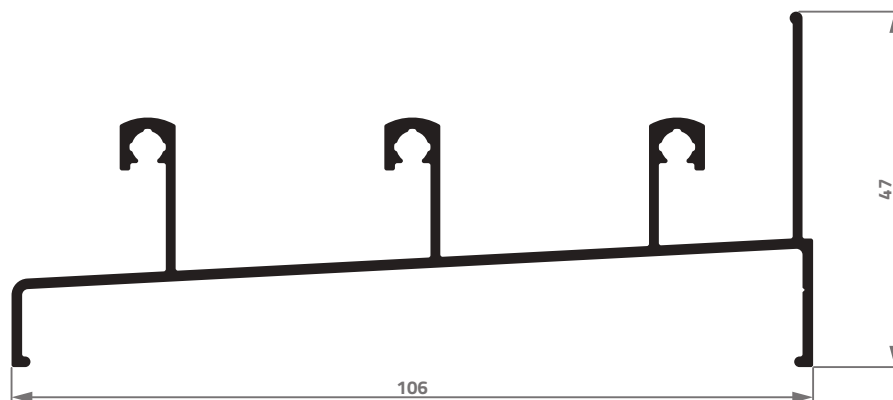
AS-011 0,967 Kg/m
