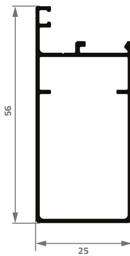
25504L 0,497 Kg/m
