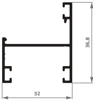
AG-068 0,369 Kg/m
