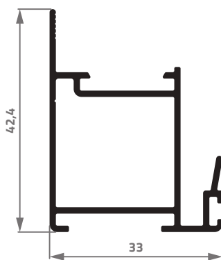
AS-041 0,506 Kg/m
