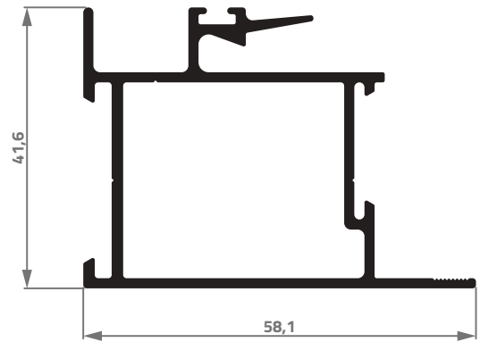
AG-049 0,905 Kg/m
