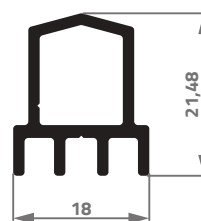
AG-061 0,320 Kg/m
