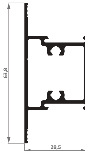
AG-055 0,756 Kg/m
