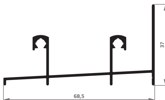
AS-228 0,609 Kg/m
