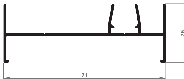
AS-003 0,490 Kg/m
