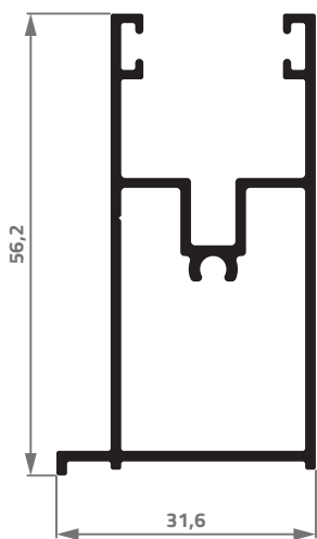
MN-007 0,705 Kg/m
