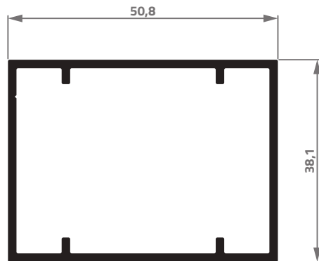
PC-004 0,795 Kg/m
