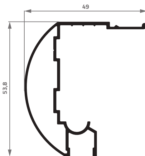
2910-BOX 0,607 Kg/m
