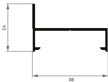
CM-060 0,269 Kg/m
