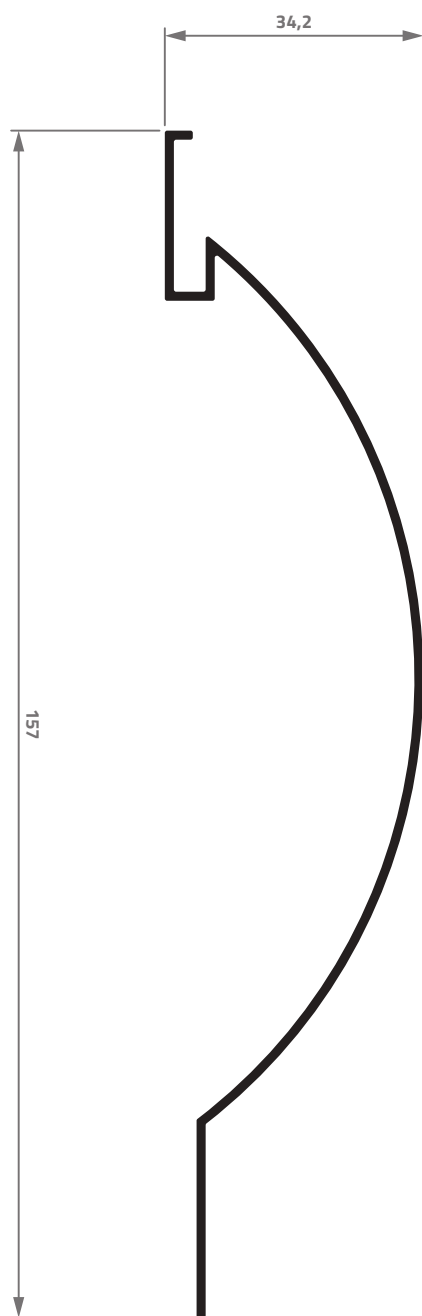
LB-002 0,638 Kg/m
