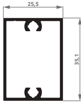
CG-012 0,501 Kg/m
