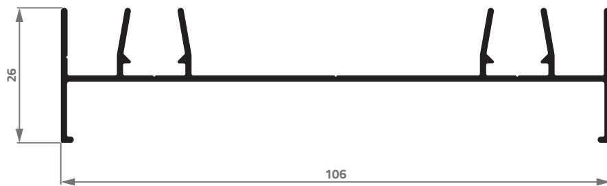
AS-013 0,707 Kg/m
