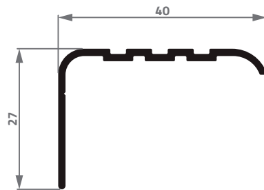
ME-013 0,267 Kg/m
