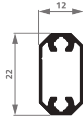
CG-022 0,238 Kg/m
