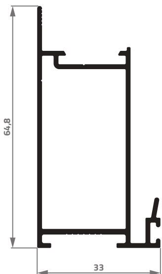
AS-242 0,712 Kg/m
