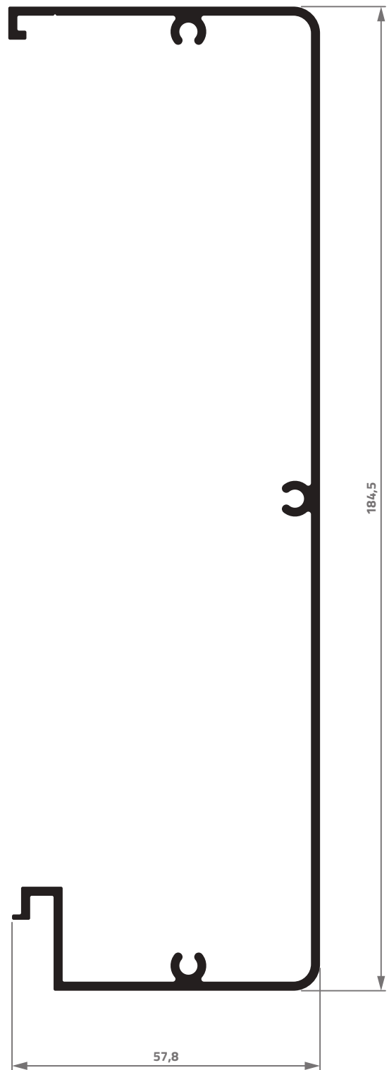
MN-032 1,653 Kg/m
