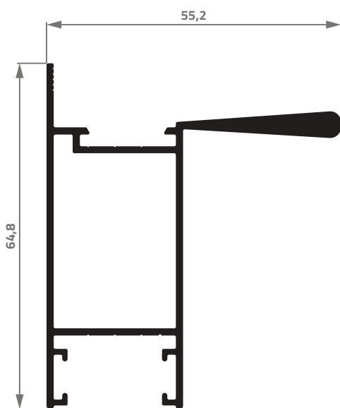
AS-280 0,915 Kg/m
