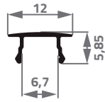
3075 0,056 Kg/m
