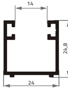
2936 0,365 Kg/m
