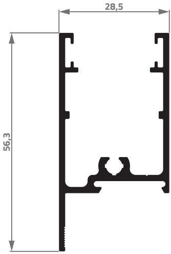
AG-006 0,675 Kg/m
