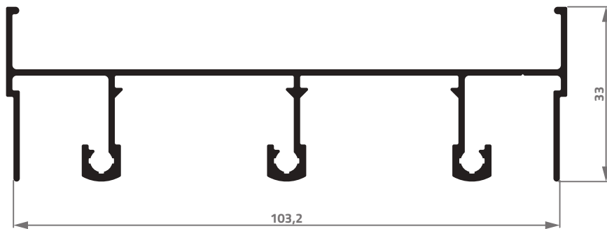
AS-010 0,970 Kg/m
