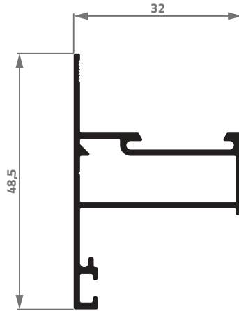
AG-085 0,466 Kg/m
