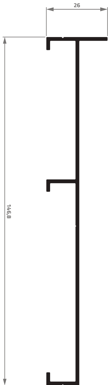
AG-158 0,897 Kg/m
