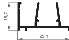
AS-008 0,247 Kg/m
