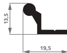
XA-247 0,191 Kg/m
