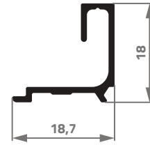
AG-027 0,149 Kg/m
