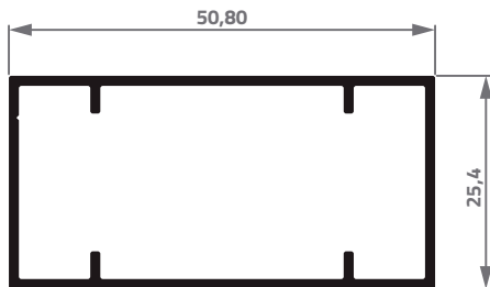
PC-002 0,520 Kg/m
