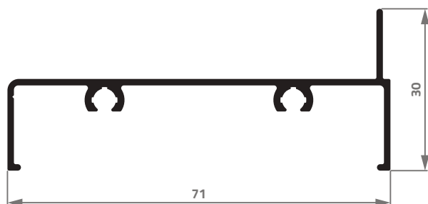
AS-004 0,479 Kg/m
