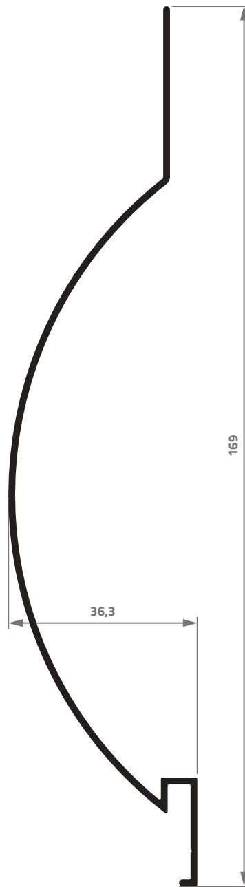
LB-002G 0,726 Kg/m
