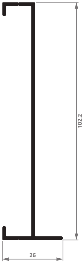
AG-002 0,639 Kg/m
