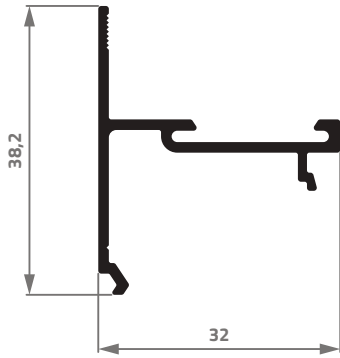
AG-077 0,327 Kg/m
