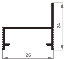
CM-200 0,200 Kg/m
